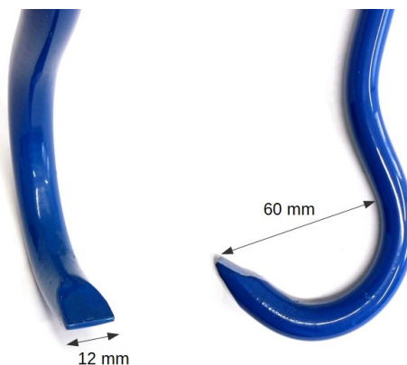
Rozměry konce háku
